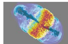
星間ガスとジェットの相互作用
