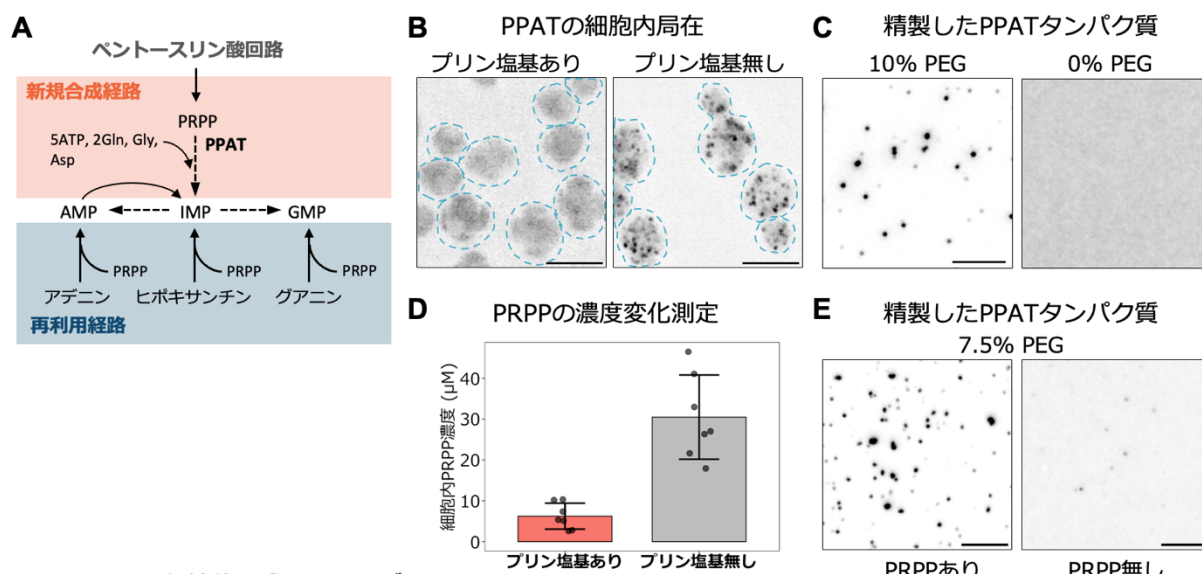
図2 PPATの凝縮体形成のメカニズム
