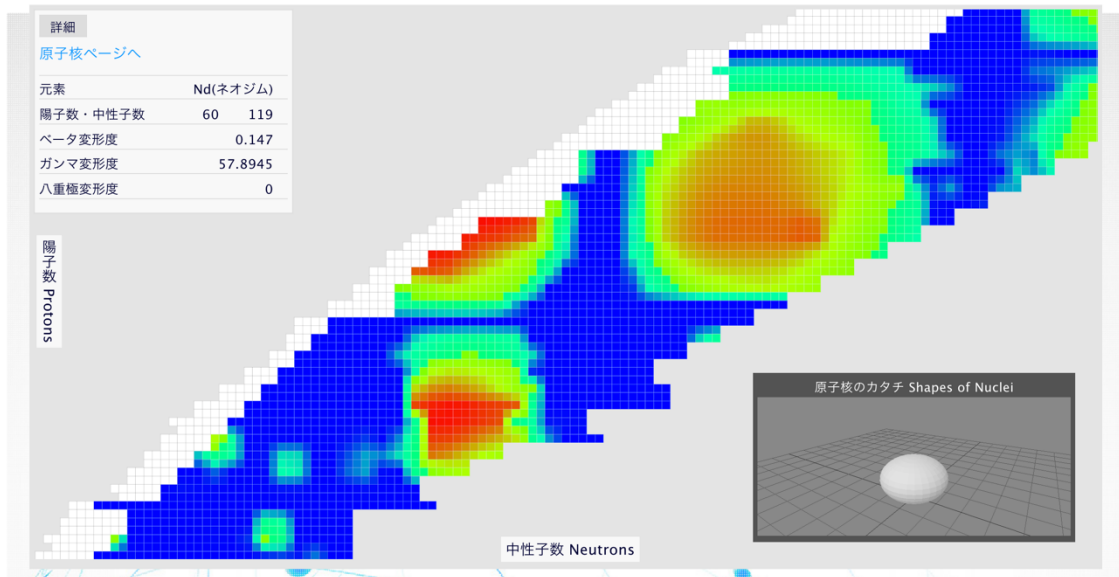
参考図 1 : ウェブサイト InPACS に公開したデータの一つ、カタチの核図表。図中の色は形の違いを表している。核図表の特定の原子核をクリックすると、その原子核の形が右下に表示され、陽子数、中性子数などが左上に表示される。原子核の形はマウスで自由に回してみることができる。
