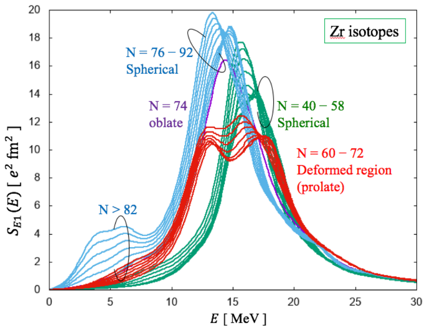
参考図 2 : ジルコニウムのアイソトープ (同位体) における光吸収断面積および中性子反応断面積を決める E1 強度関数の計算核データ (横軸は光 (フォトン) のエネルギー)。中性子数の変化に応じて、原子核の形が球形 (緑)、プロレート型 (赤)、オブレート型 (紫) と変化することで、E1 強度関数の様相が大きく変化する。また、中性子数が 82 を越えた領域 (水色) では、低エネルギーに E1 強度の増加が見られる。この中で実験データが存在する核種は、 ^{90, 91, 92, 93, 94, 96}\text{Zr} の 5 核種のみである。
