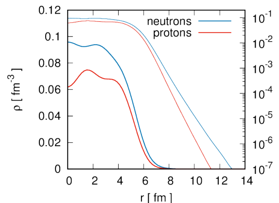
参考図 3 : LLFP の一つ ^{107}\text{Pd} の原子核に対する公開した計算核データの一例。左の表には、基底状態における形の情報、半径の大きさ、超流動性の指標であるギャップエネルギー、1 核子分離エネルギーの逆符号に対応する化学ポテンシャルが示されている。右図は陽子・中性子の密度分布を原子核中心からの距離の関数として表示。
