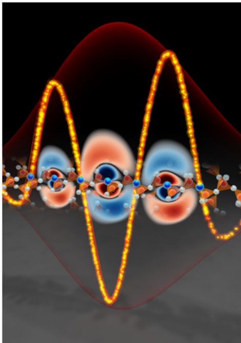
図：左から来る黄色い光が二酸化ケイ素の原子に照射し、各原子の周りにはいる電子を振動させる。この電子の動きが光波のエネルギーを吸収する。パルス光の終わり、電子による吸収されたエネルギーは再び光波に戻る。この物質を通過した後の光波の時間波形を正確に測定し、アト秒の速さで変化する固体の電子の運動を、実時間観測することが可能になった。
