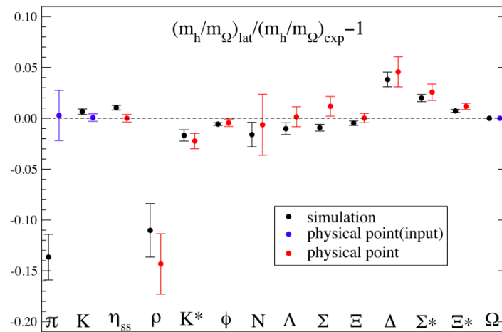
図1 ハドロン質量の実験値との比較
