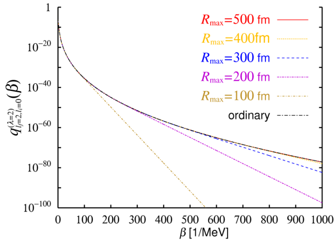
図4: \alpha - ^{16}\text{O} 光捕獲反応率に対する計算。通常の計算法 (ordinary) と、様々な空間領域で得られた虚時間計算法との結果を比較している。この系では、500fm の空間で解くことにより、1000MeV ^{-1} (10 ^7 K 程度) の温度領域まで収束した結果が得られている。
